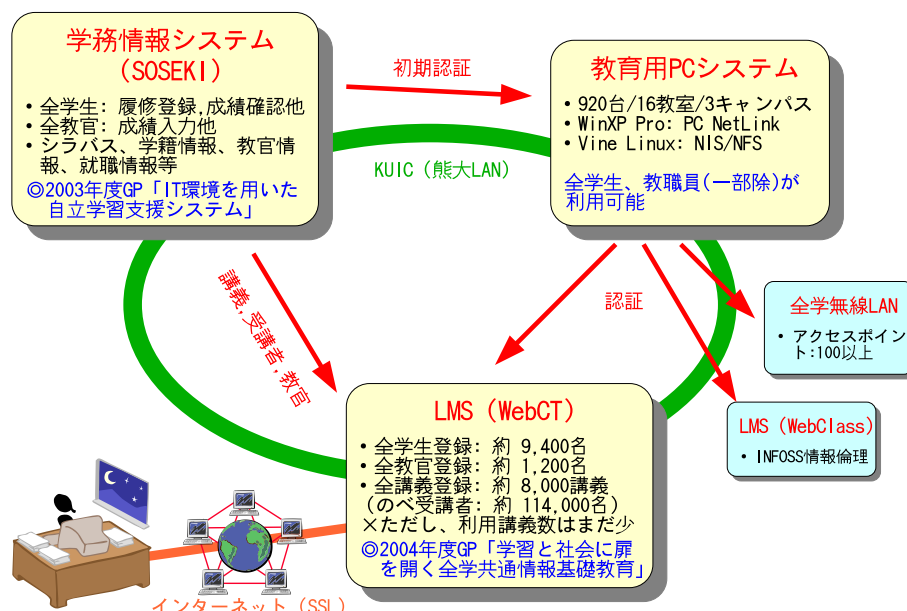
図 1: システム間データ連携の概念図
